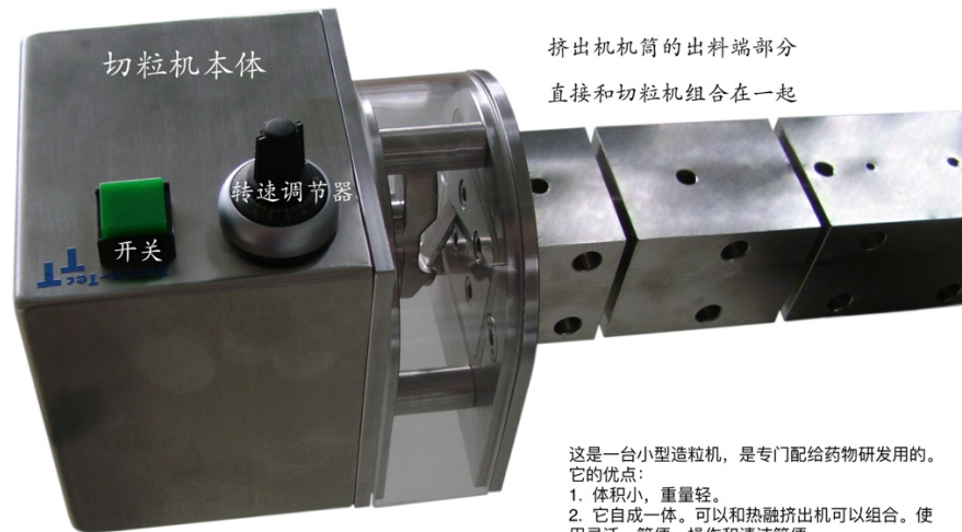
小型切粒机
